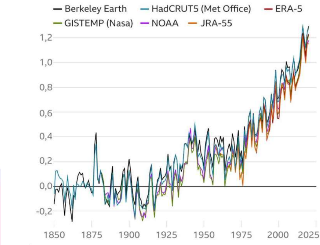
Gráfico 2.1 Incremento de temperatura media global desde 1850
